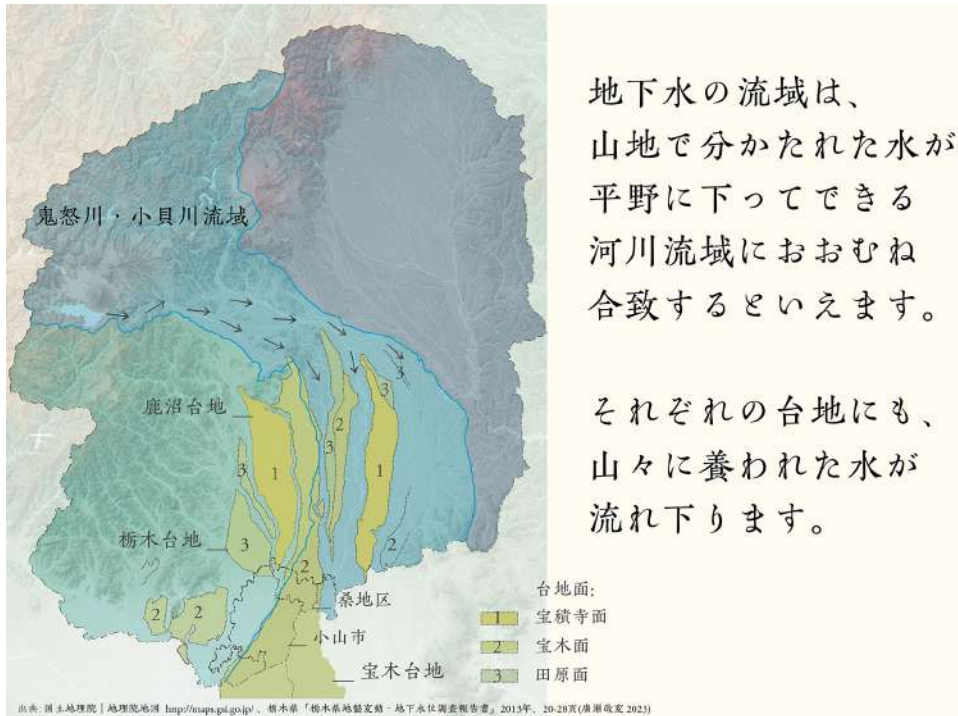
図 10 栃木県の河川流域圏と小山市周辺の台地の分布
