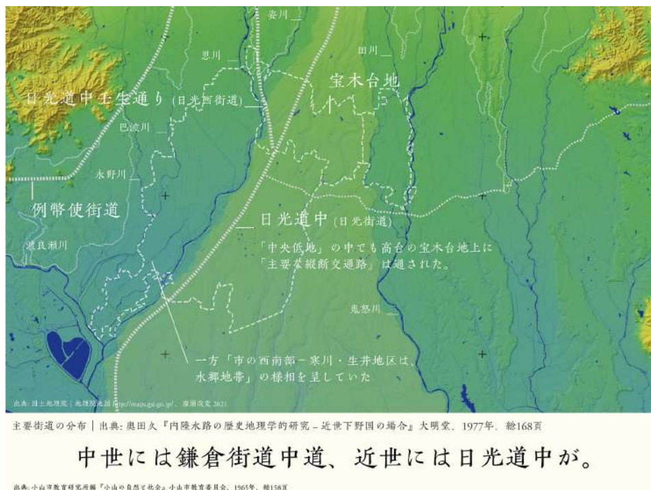
図23 小山市周辺の地形に主要街道の分布を重ねる。
