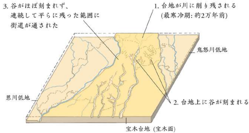
台地上での侵食谷の発達過程を表わした概念図 (廣瀬 2023) *
