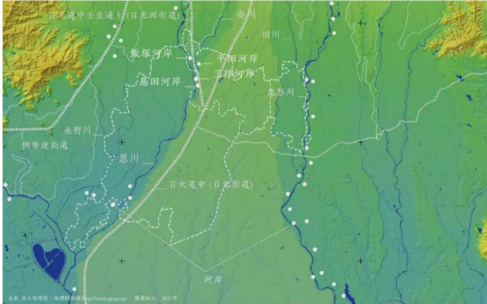
渡良瀬川、巴波川、思川、鬼怒川の河岸の分布 | 出典1: 奥田久監修『栃木の水路』栃木県文化協会、1979年、総376頁
