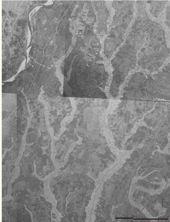
図8 空中写真(1974年撮影)を用いて当地区の地形を見る。色の薄い樹枝状の箇所が谷。
